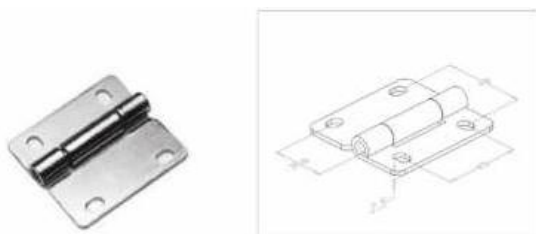
Balama intermediară
