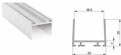
Profil aluminiu
