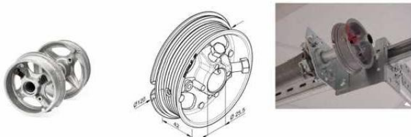
Tambur
