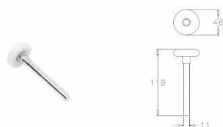
Rolă
