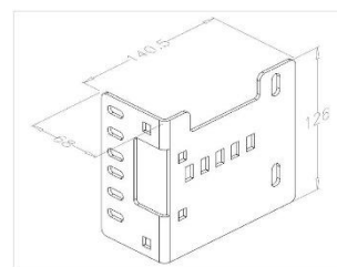
Suport ax lateral
