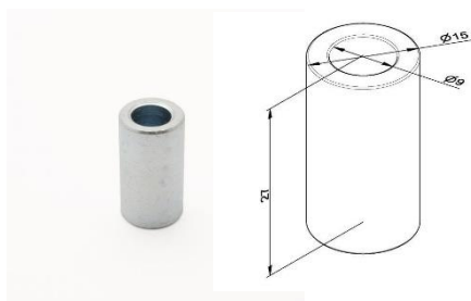
Inel distanțier șină joasă
