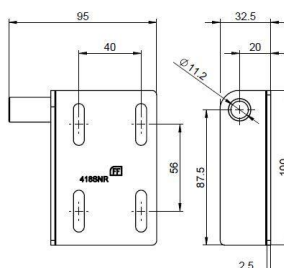
Balama superioară
