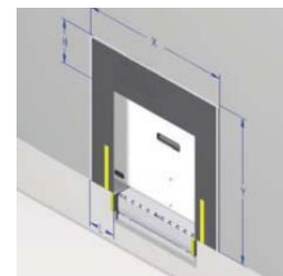
Structura burdifului de fațadă
